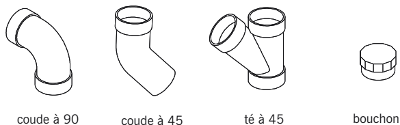
fig. 19.3 raccords
